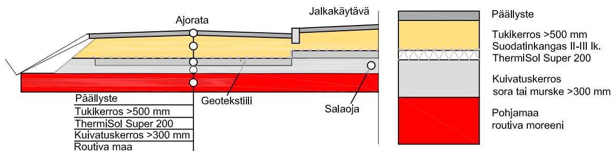
Routaeristetty katupoikkileikkaus
