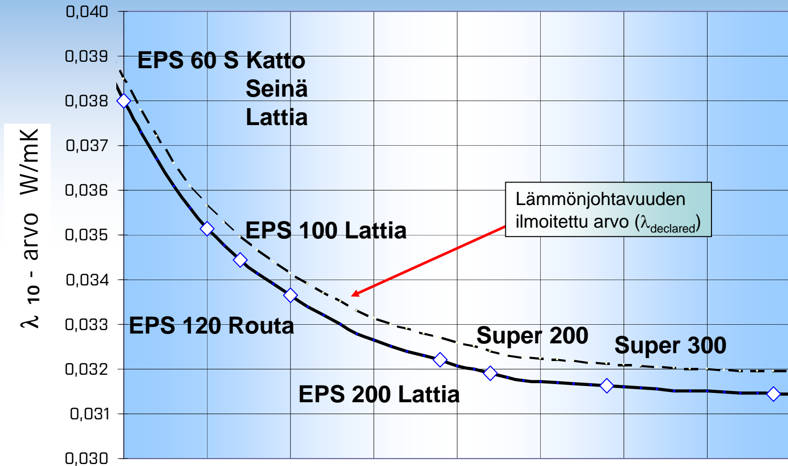
Lämmönjohtavuuden riippuvuus lujuusluokasta
